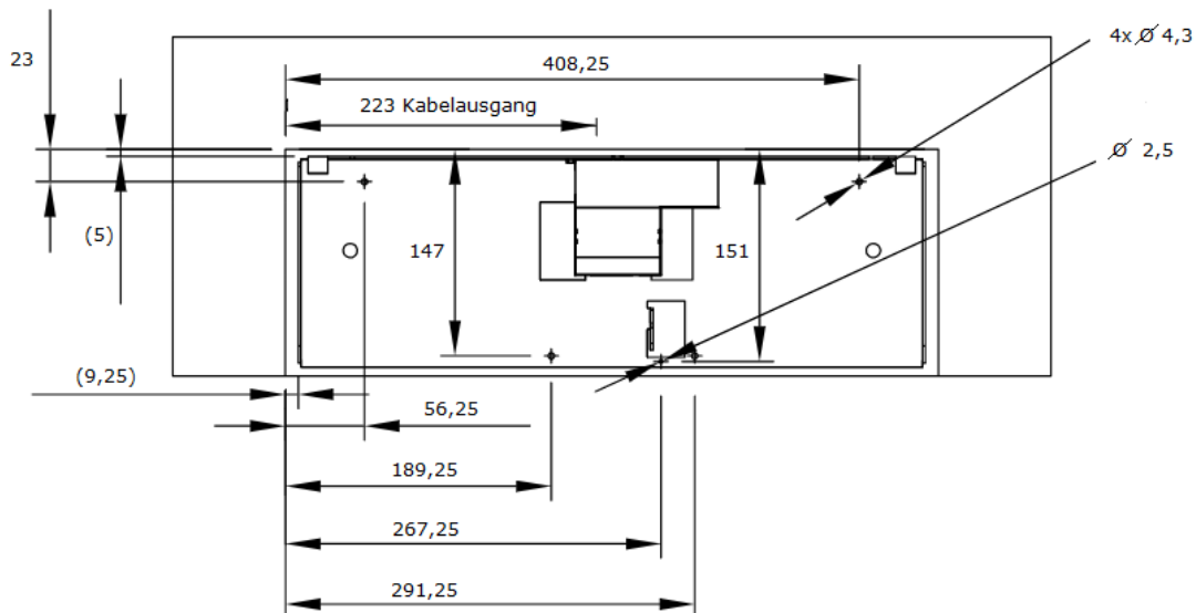
Befestigungslöcher für die Bodenplatte
